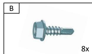
Sraigtas DIN 7504 K 6,3x19
