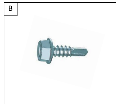
Sraigtas/Screw DIN 7504K 6,3x19
